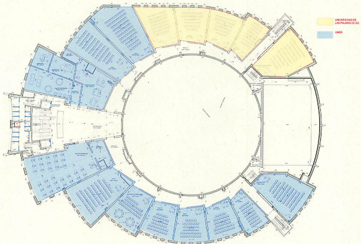
Planta tercera
