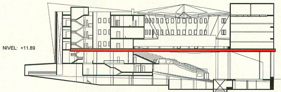
Sección longitudinal
